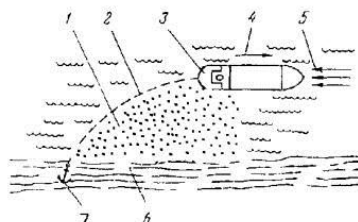
Рис. 18. Перемещение судна для увеличения ограждаемого судном и бонами участка: 1 - нефтяное пятно; 2 - оперативные боновые заграждения; 3 - аварийное судно; 4 - направление передвижения судна; 5 - направление течения; 6 - линия берега; 7 - якорь
