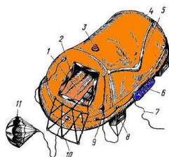
Рис. 9 Устройство надувного спасательного плота 1 – надувное днище; 2 – шторы входа; 3 – сигнальный огонь; 4 – двойной тент; 5 – водосборник; 6 – газовый баллон; 7 – пусковой линь; 8 – водобалластный карман; 9 – леер; 10 – входной трап; 11 – плавучий якорь
