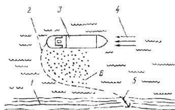
Рис. 17. Предотвращение растекания нефти корпусом судна и боковыми заграждениями: 1 - линия берега; 2 - оперативные боновые заграждения; 3 - аварийное судно; 4 - направление течения; 5 - якорь; 6 - нефтяное пятно
