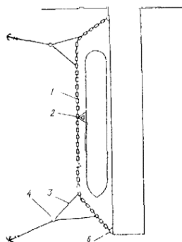
Рис. 16. Ограждение бонами судна, стоящего у причала: 1 - боновое заграждение; 2 - треугольная распорка из досок; 3 - капроновая оттяжка; 4 - буй на якорю; 5 - узел крепления к причалу
