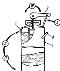
Рис. 13. Пенный огнетушитель.
