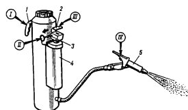
Рис.15. Порошковый огнетушитель.
