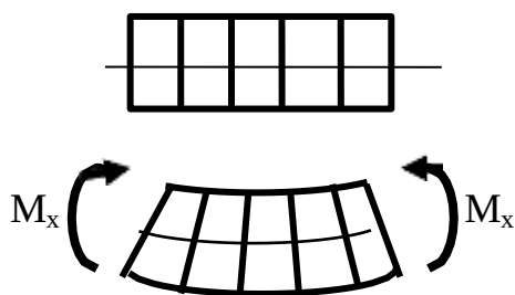
Гипотеза Бернулли.
